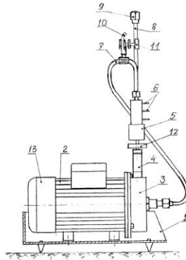
Рис. 1. Принципиальная схема гидродинамического контура с кавитирующим соплом.
