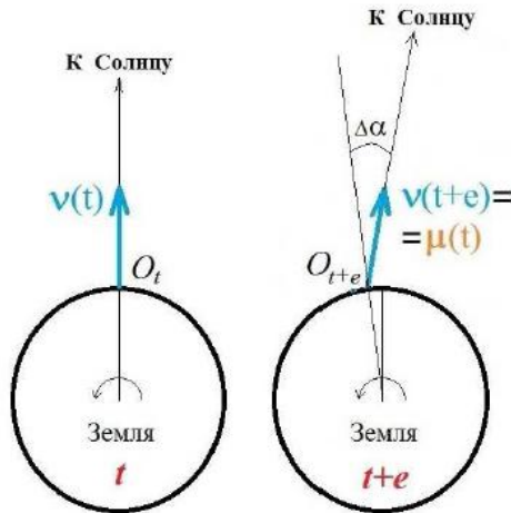
Рис. 1. Направления на Солнце для наблюдателя O в моменты t и t + e .
