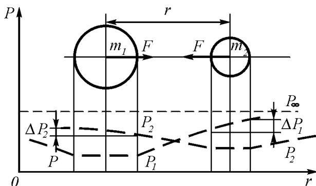
Рис. 3.1. Механизм гравитационного взаимодействия тел: изменение температуры и давления эфира вблизи гравитационной массы и гравитационное взаимодействие двух масс
