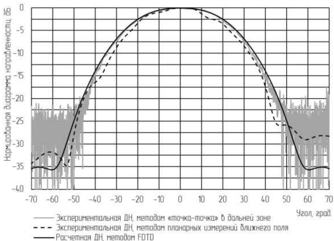
Рис.10. Сечения ДН в H-плоскости на частоте 14 ГГц, полученные различными методами
