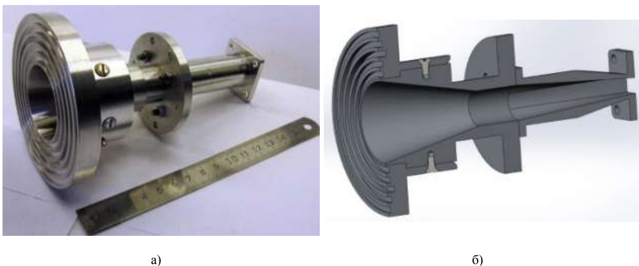
Рис. 4. Облучателя зеркала радиоколлиматора АКК1-05: после сборки (а), трехмерная модель в разрезе (б)
