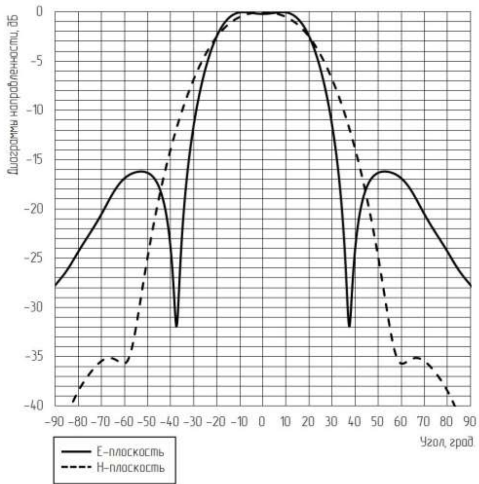
Рис. 5. Сечения нормированной диаграммы облучателя в E и H-плоскостях на частоте 14 ГГц
