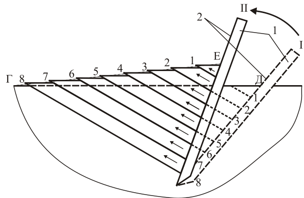
Рис. 2. Схема разрушения грунта при работе анкерного устройства [10]: 1 – рабочий элемент; 2 – передняя поверхность рабочего элемента
