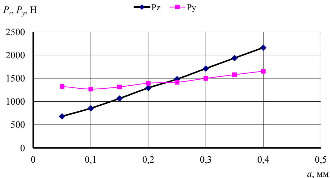
Рис. 6. Влияние толщины среза на суммарные составляющие силы резания
