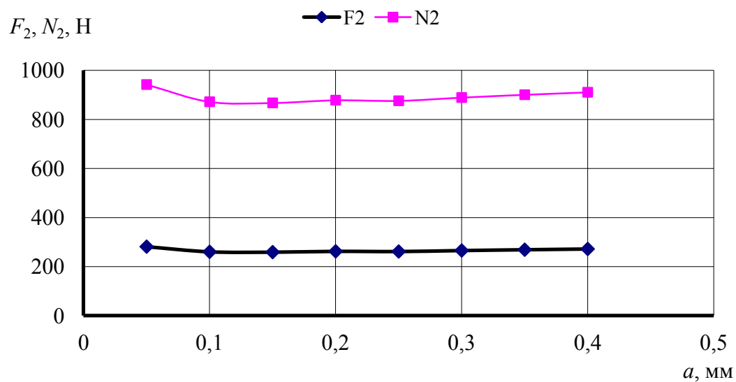
Рис. 5. Влияние толщины среза на силы на задней поверхности
