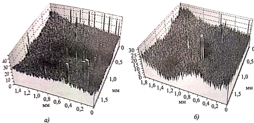
Рис. 7. Топограммы обработанных оптических поверхностей: а — ситалла CO115M; б — кварцевого стекла КУ1
