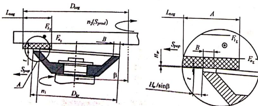
Рис. 5. Схема алмазного шлифования с наклоном оси круга
