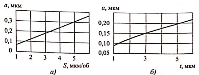
Рис. 1. Зависимость толщины срезаемого слоя: а — от подачи заготовки; б — от глубины резания
