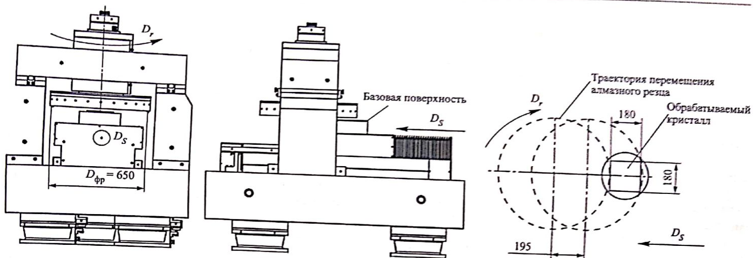
Рис. 2. Кинематическая схема обработки на сверхточном экспериментальном стенде для алмазного микрофрезерования
