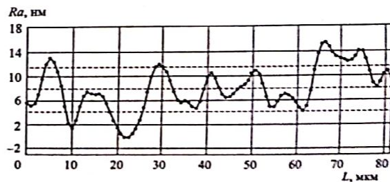
Рис. 3. Профилограмма обработанной поверхности заготовки из KDP
