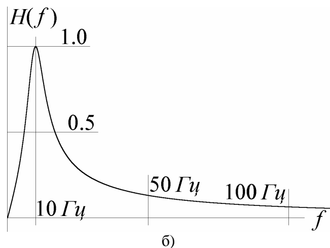
Рис.17. Расположение нулей и полюсов передаточной характеристики фильтра рис.16 (а) и его амплитудно-частотная характеристика (б)
