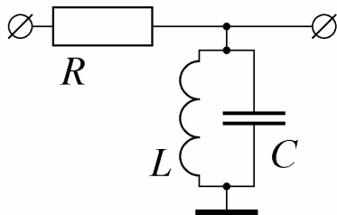
Рис.16. Непрерывная цепь второго порядка.
