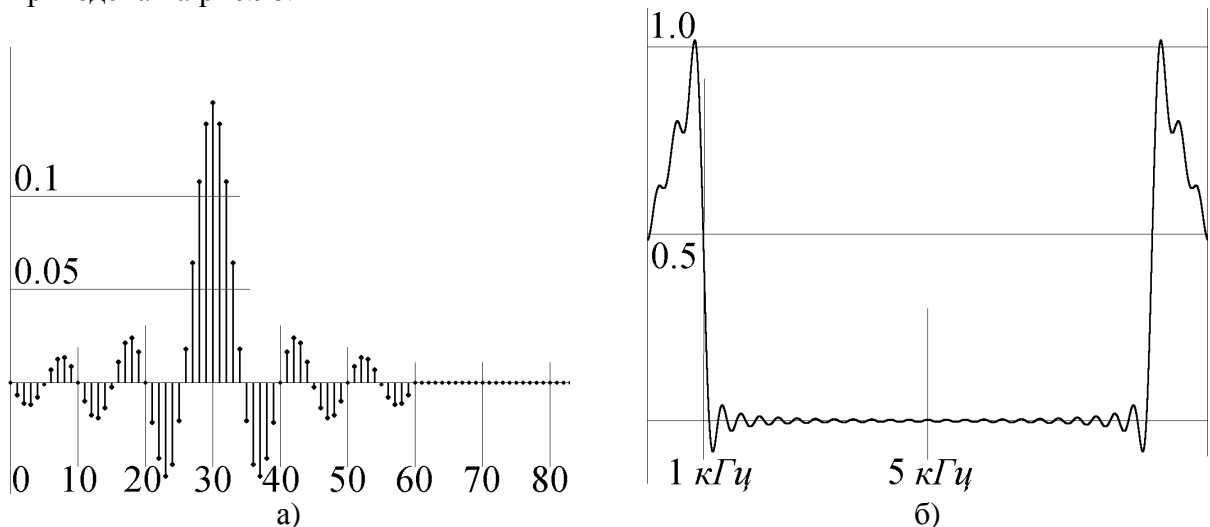
Рис.9. Импульсная и частотная характеристики цифрового фильтра примера 8, полученные после применения прямоугольного окна шириной 61.
