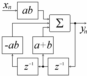
Рис.5а. Фильтр с передаточной характеристикой, содержащей два полюса.
