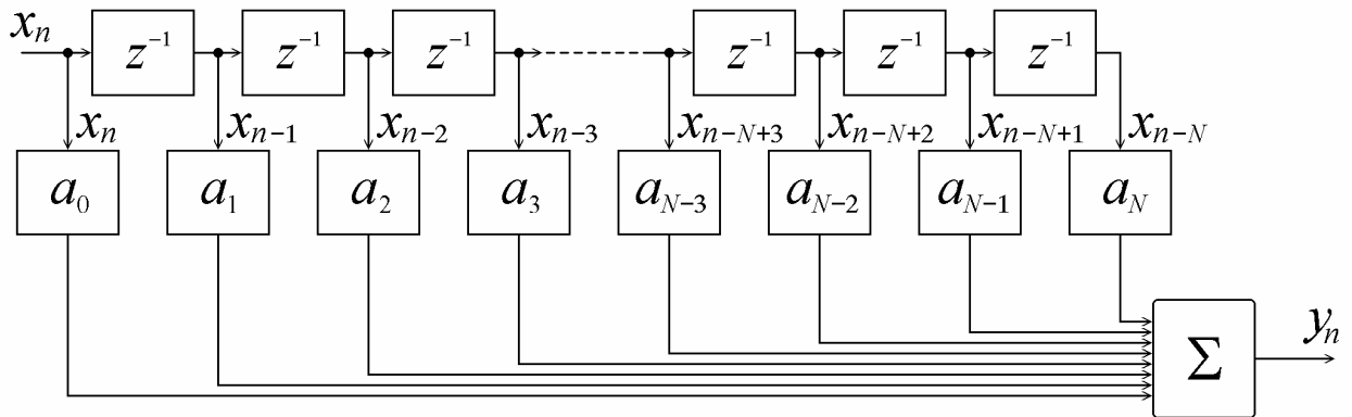
Рис.3. Структурная схема трансерсального цифрового фильтра.
