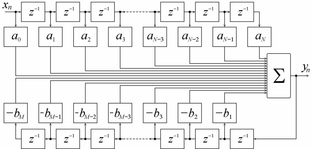
Рис.6. Первая прямая форма построения цифровых фильтров.
