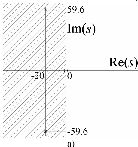
Рис.17. Расположение нулей и полюсов передаточной характеристики фильтра рис.16 (а) и его амплитудно-частотная характеристика (б)
