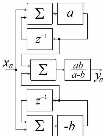
Рис.5в. Параллельное соединение фильтров первого порядка.
