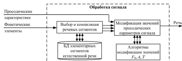
Рис. 4. Схема конкатенативного метода генерации речевого сигнала
