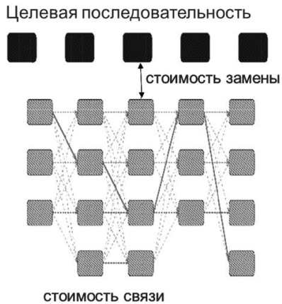
Рис. 7. Оптимальной выбор звуковой последовательности (UNIT SELECTION)
