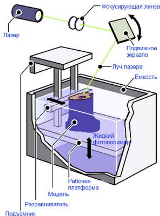
Изображение №1. SLA технология.
