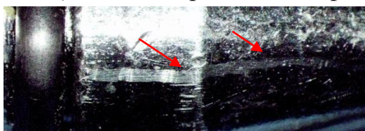
Рис. 7. Фрагмент стержня с двух сторон с первичными следами (показаны красителем красного цвета) от фигурной цанги
