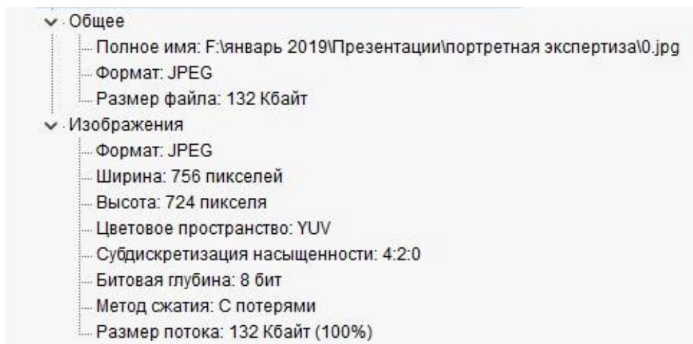
Рис. 1. Технические сведения, полученные посредством использования программы «MediaInfo»
